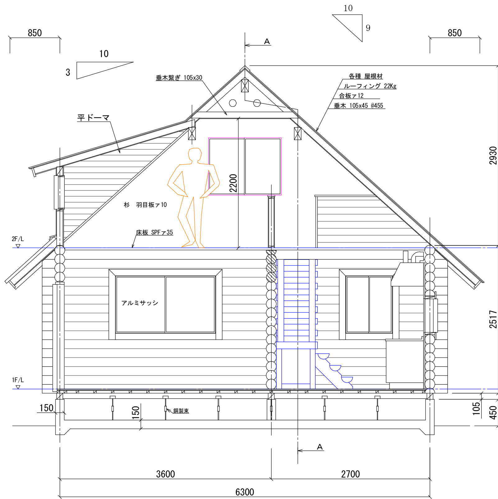
正面矩計図
